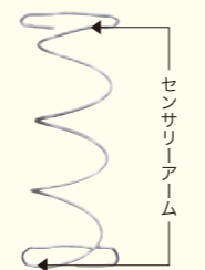
線径2mm・5巻・コイル高145mm
